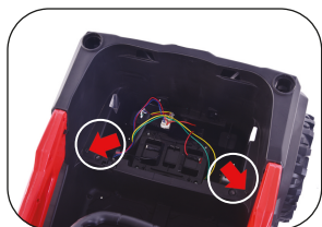
5.6 Retire los tornillos de la zona del asiento, colocados en sus extremos.
