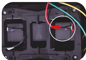
4.2 Conecte el cable rojo al extremo rojo de la batería.
